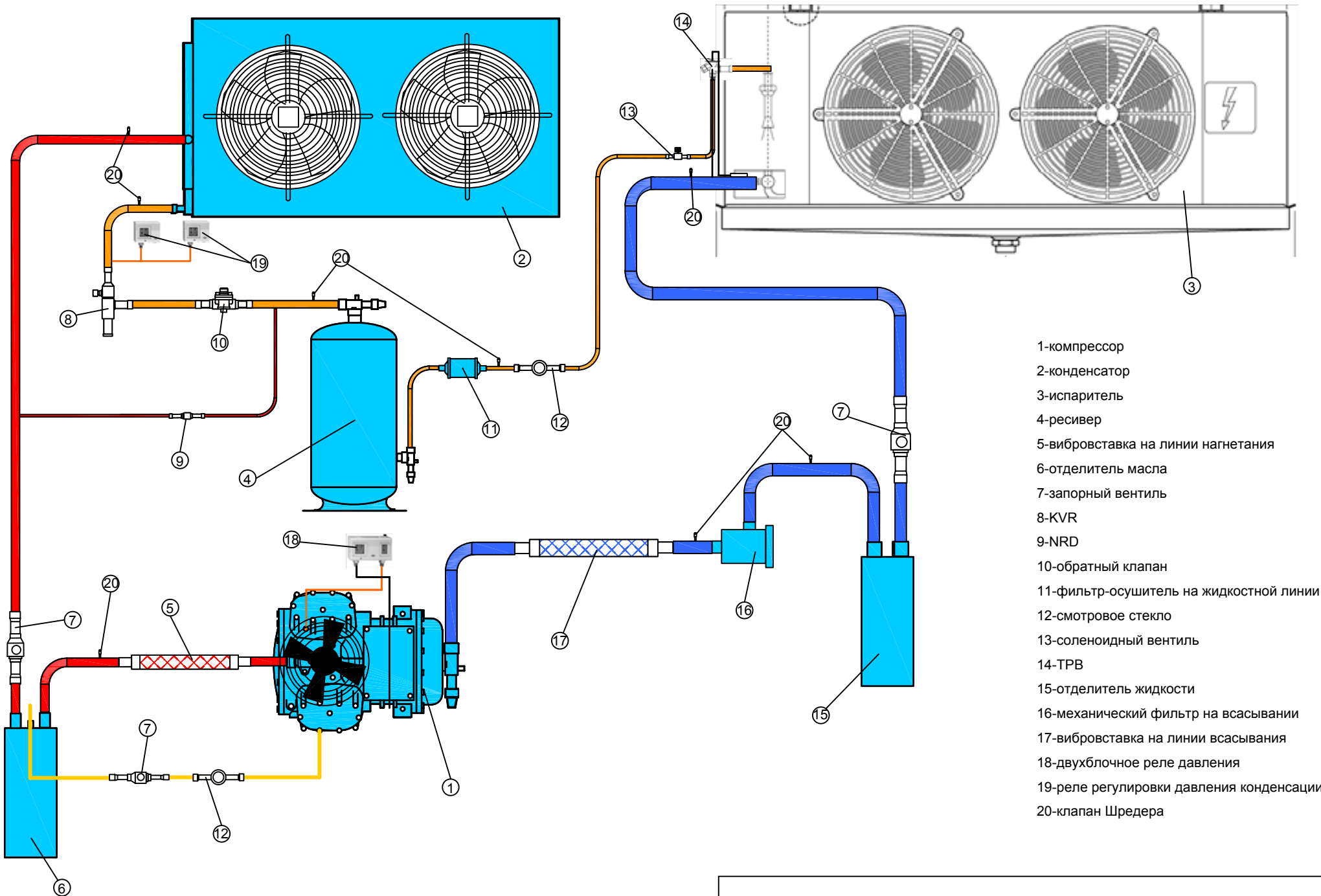
Базовая структурная схема холодильной установки
